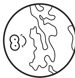
TITAN
