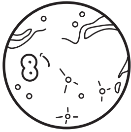
TITANIA
