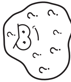
NESO
