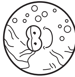
ENCELADUS
