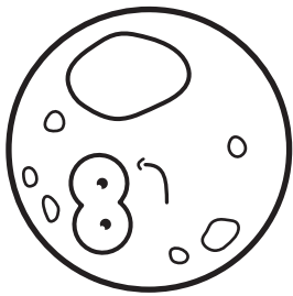
MIMAS
